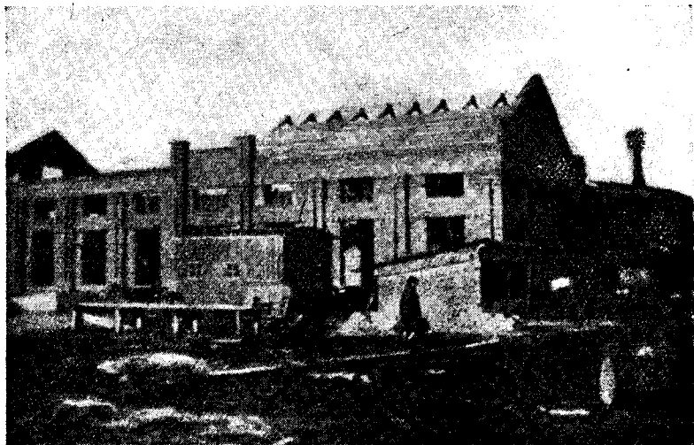
Строительство литейного цеха завода «Молот»
